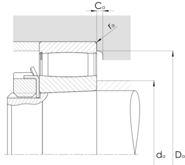
Anschlussmaße
